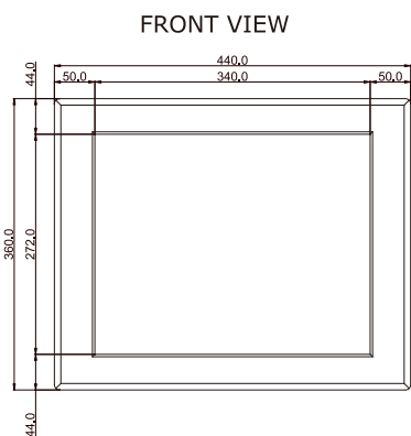
IP65 (8 mm front bezel)
