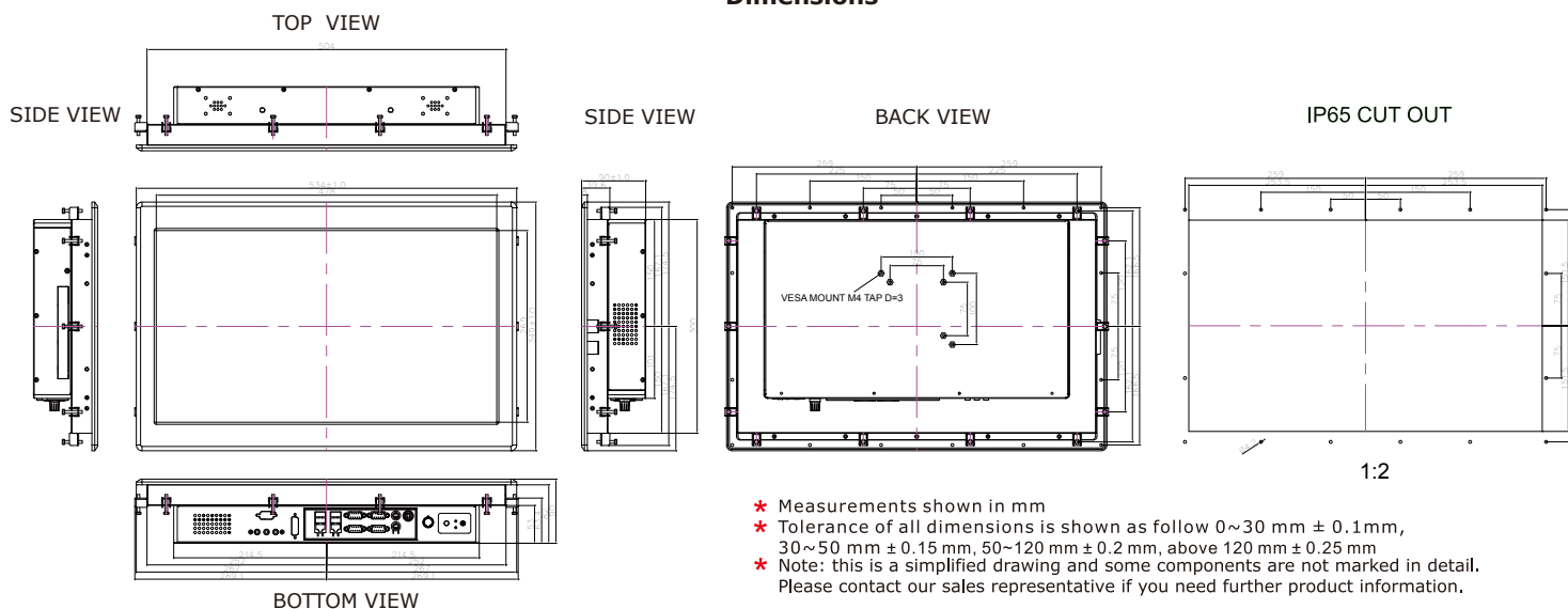
Dimensions
