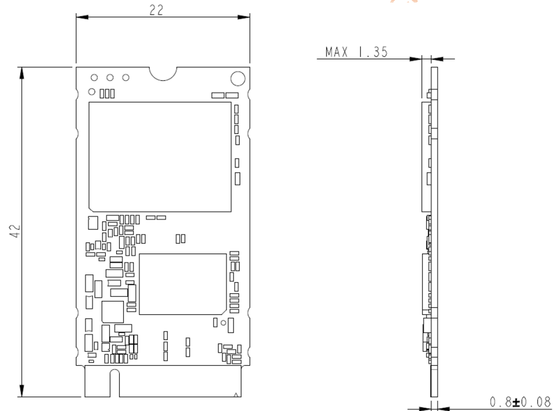
M.2 2242
