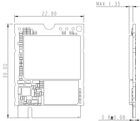
M.2 2230
